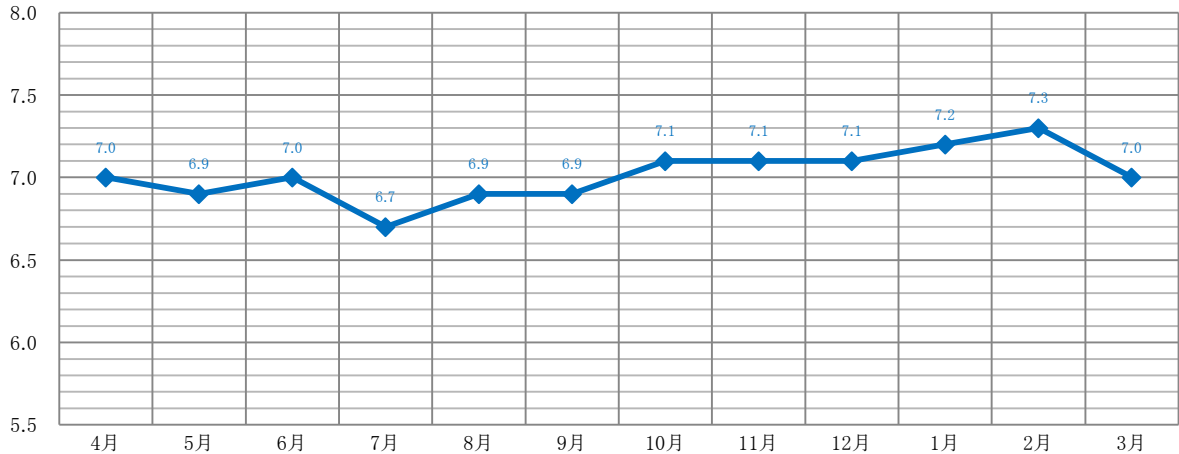
処理水月別平均pH値
